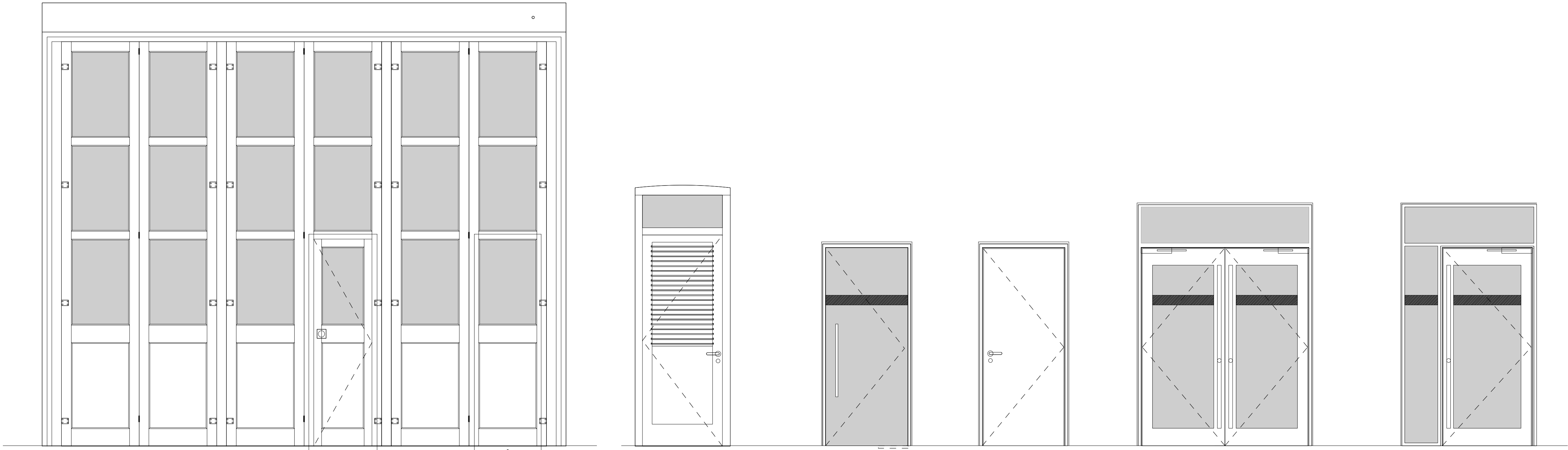
DOOR TYPE 12 SCALE 1:25 L20251 & L20.330A
