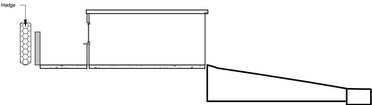
1 Existing Section 1 1 : 100
