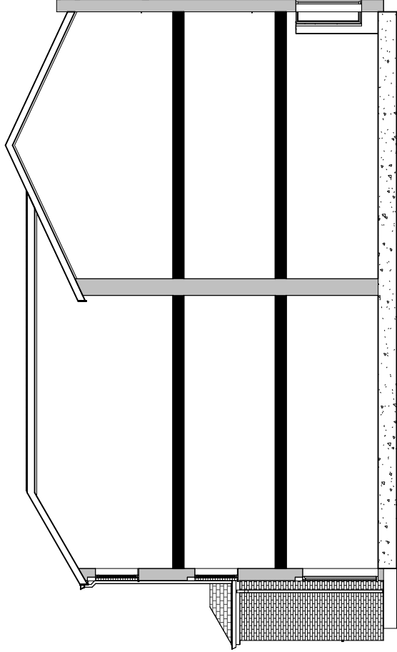
④ Existing Section 1 : 100
