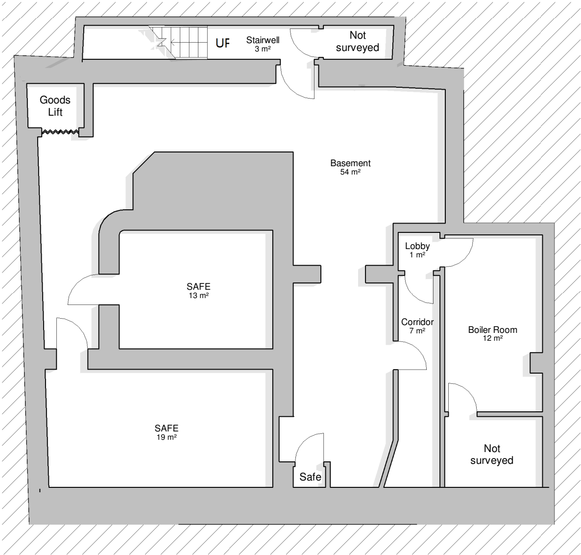
Basement 1 : 100
