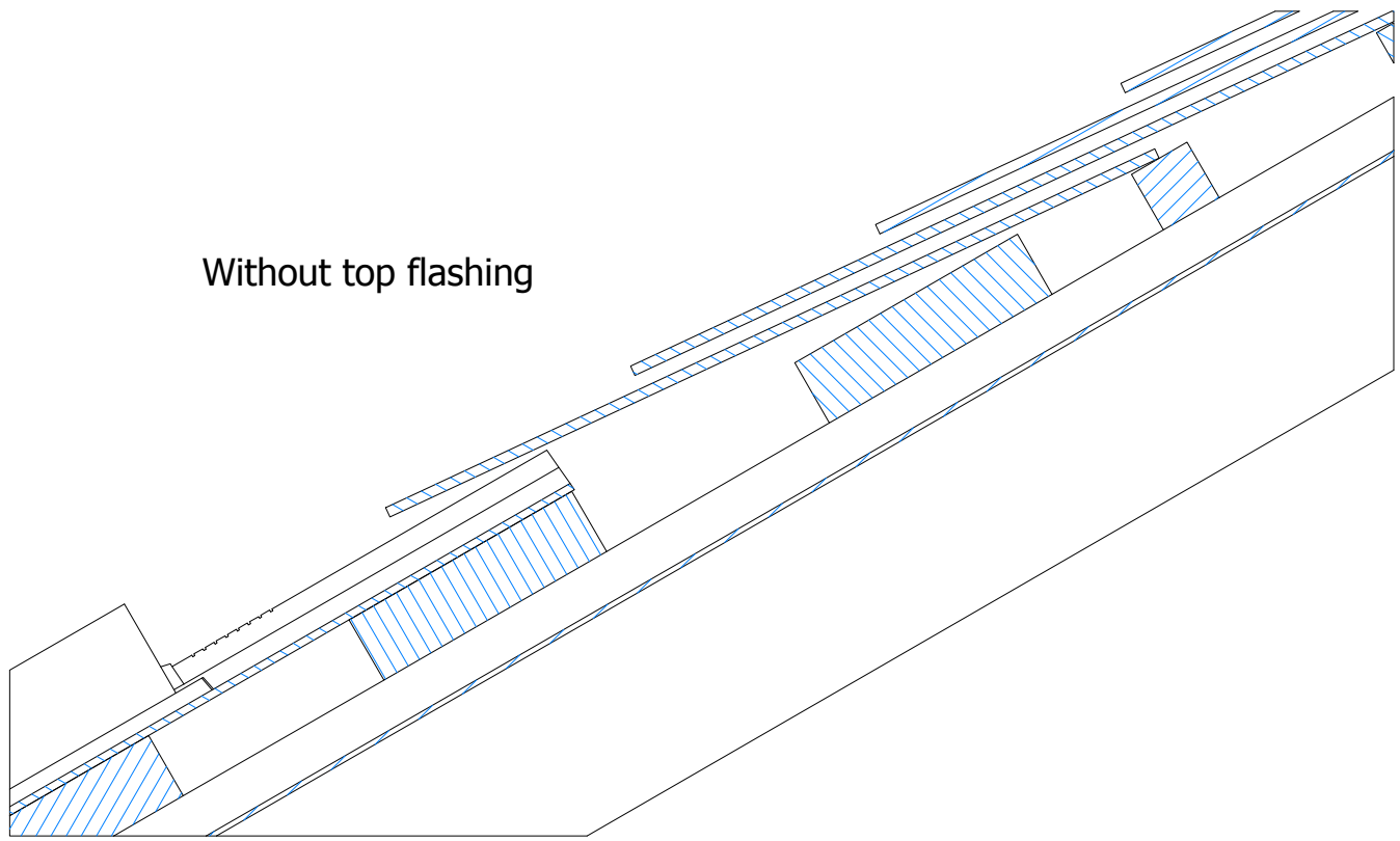
J ( 1 : 3 )
