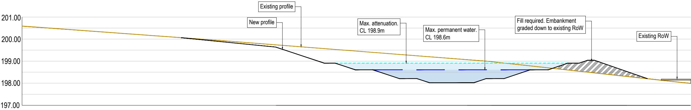
Section A-B
