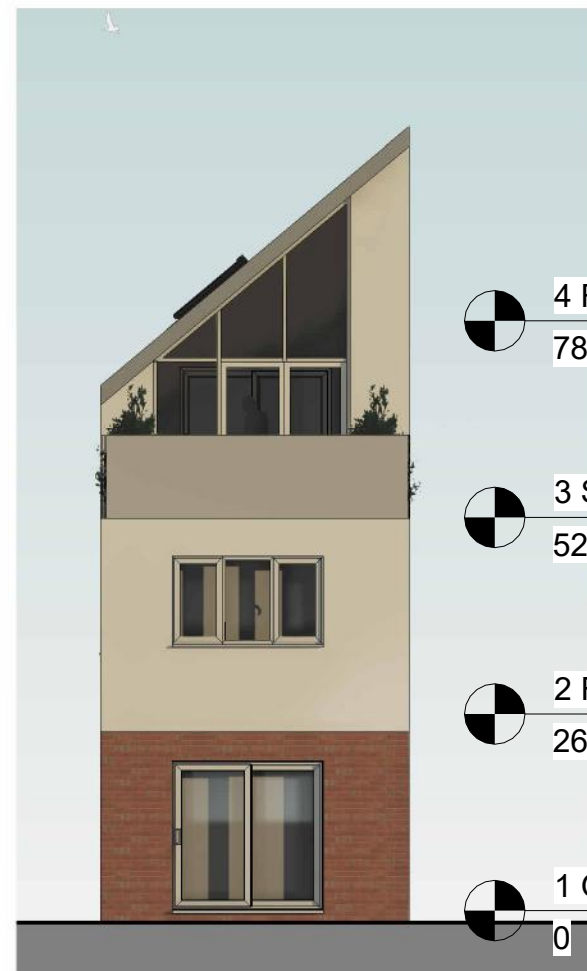
ELEVATION 1 1 : 100
