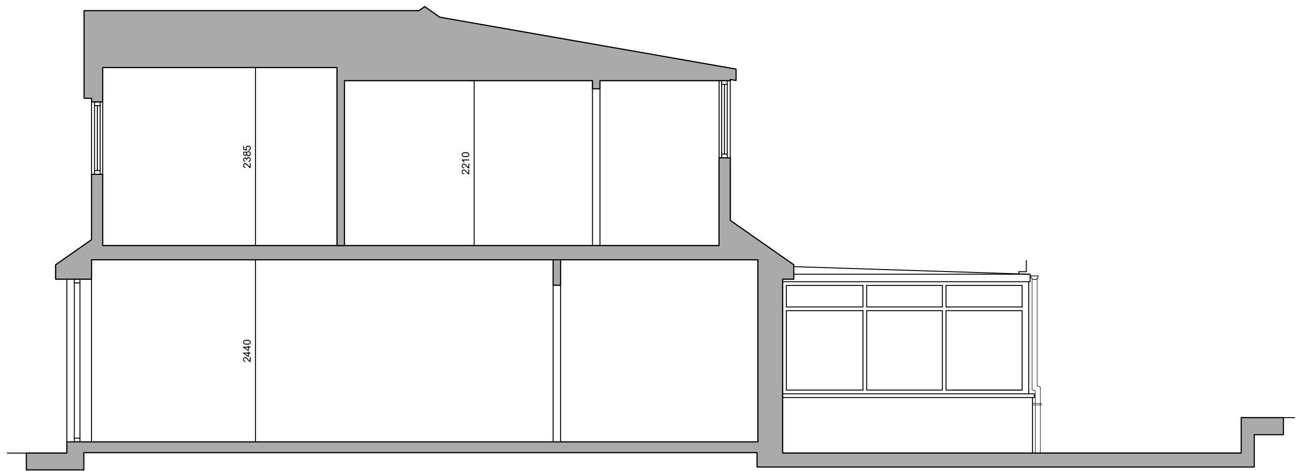
SECTION A-A
