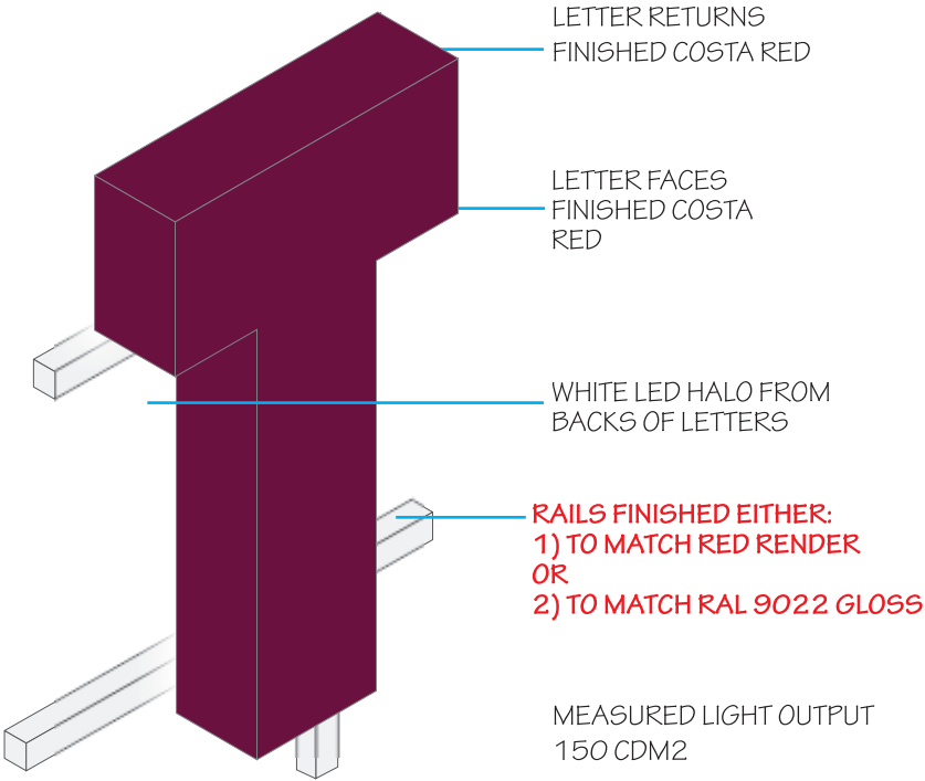
'COSTA' DETAIL
