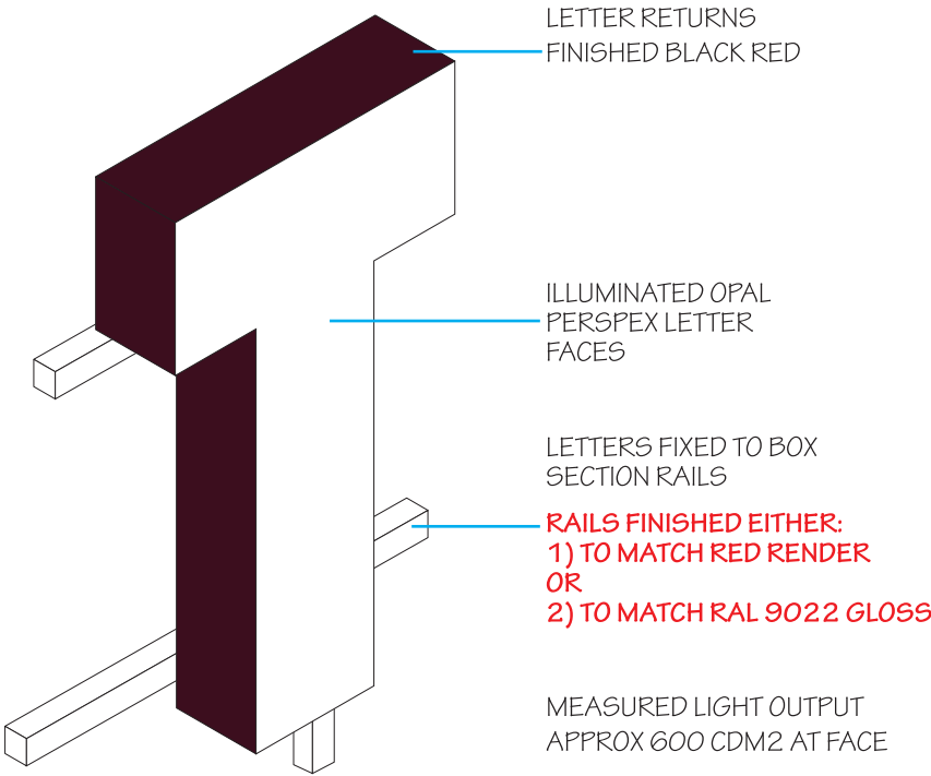
'COSTA' DETAIL
