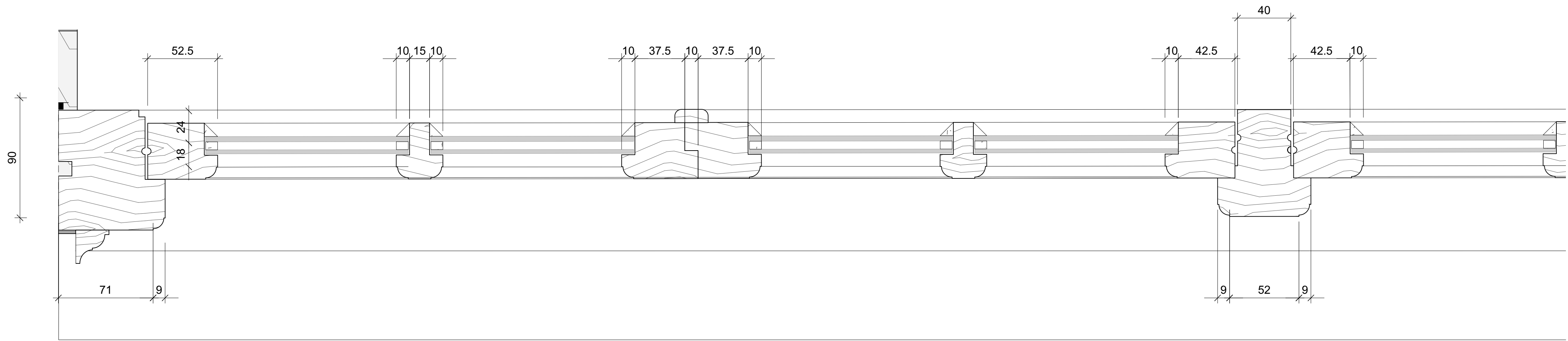
A 707.1 - JAMB SCALE 1:2
