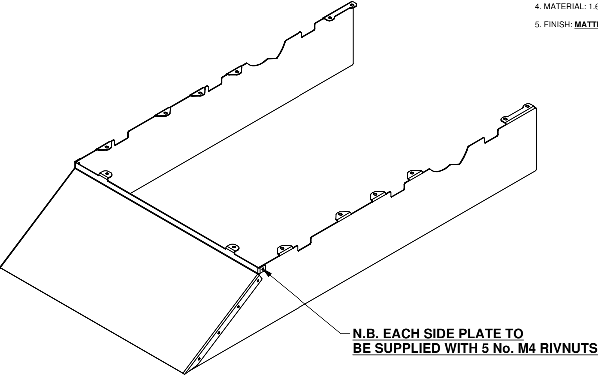
ISO (SCALE 1 : 8 )
