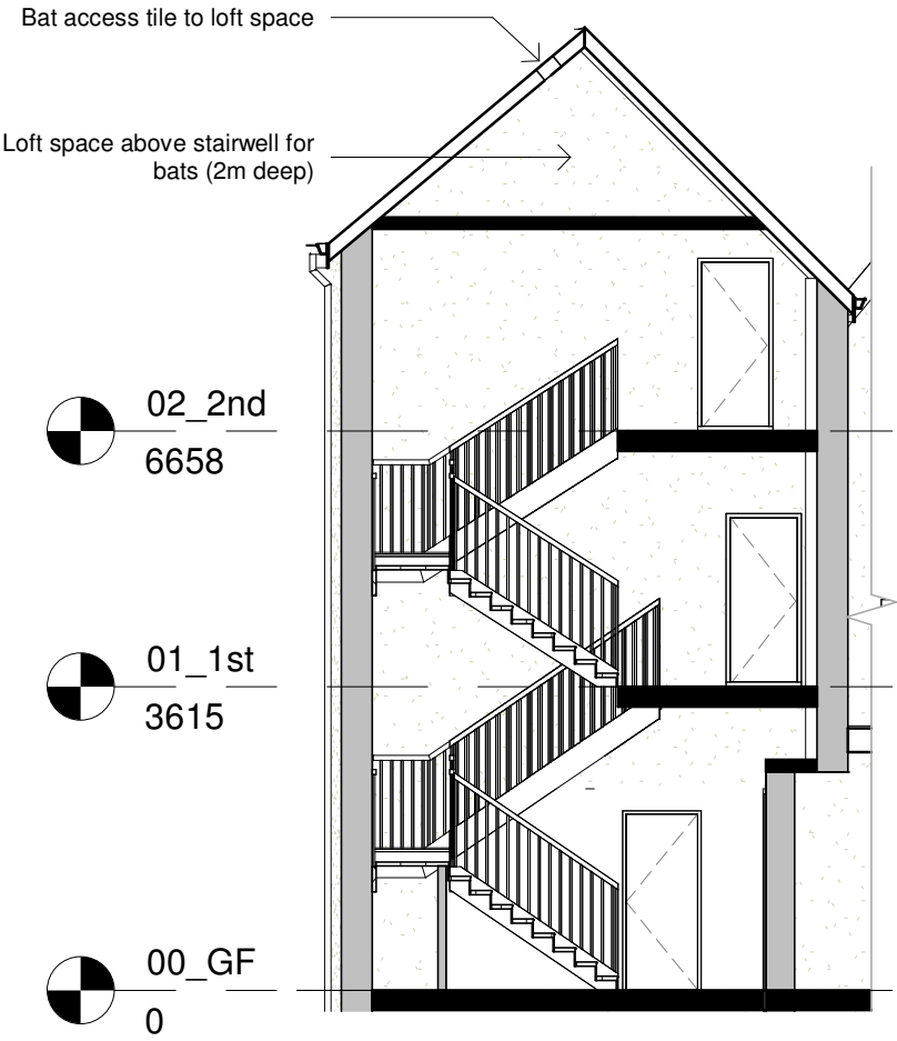
Section A - A 1 : 100
