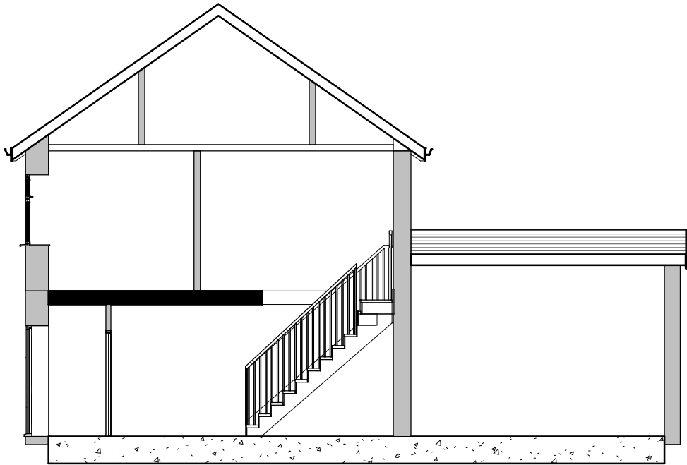
4 Existing Section 1 : 100
