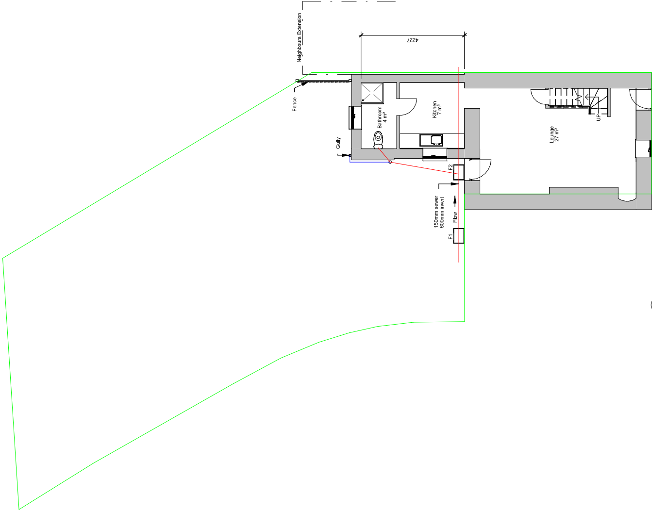
1 Existing Drain Plan 1 : 100
