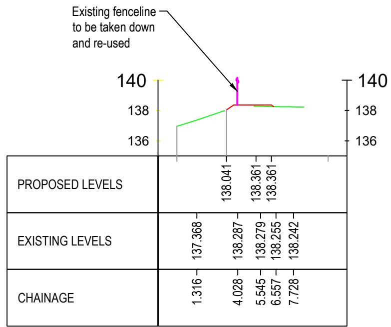
Chainage 86 SCALE: H 1:250, V 1:250
