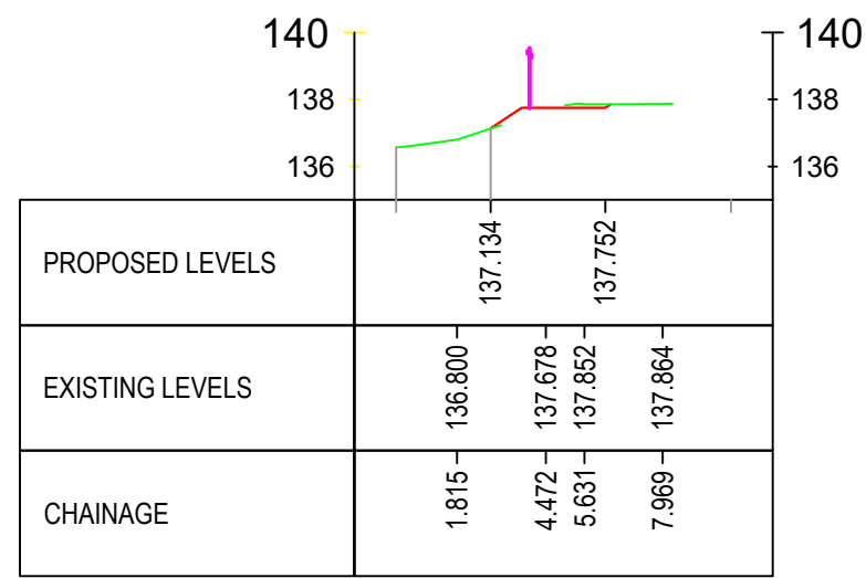
Chainage 134 SCALE: H 1:250, V 1:250
