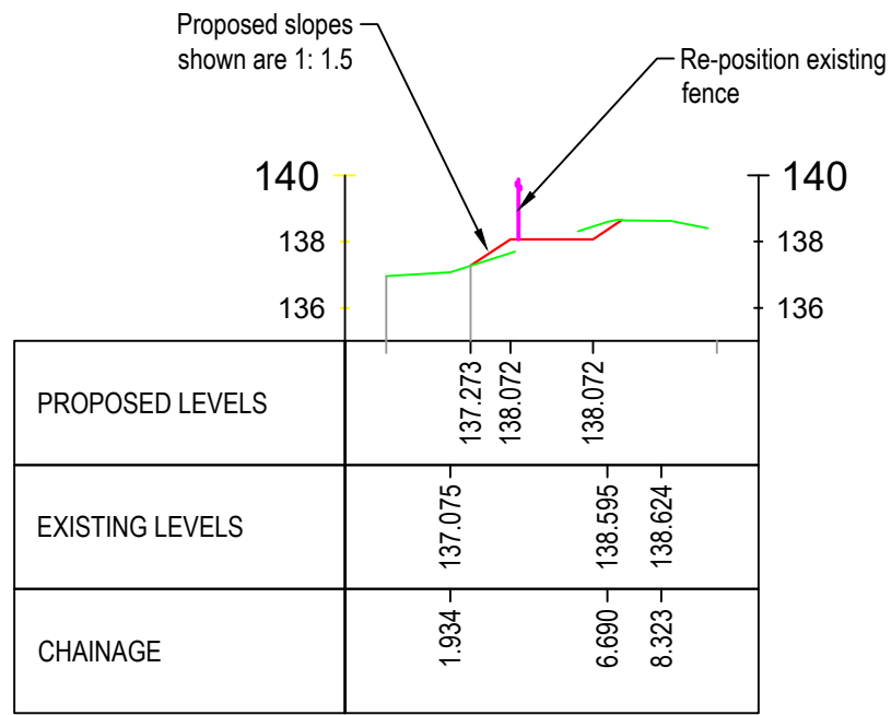
Chainage 20 SCALE: H 1:250, V 1:250
