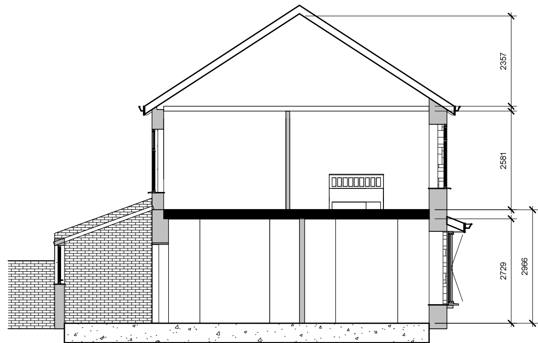
1 Existing Section 1 : 100
