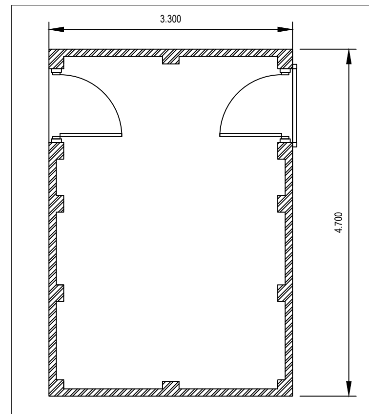
Plan 1:50
