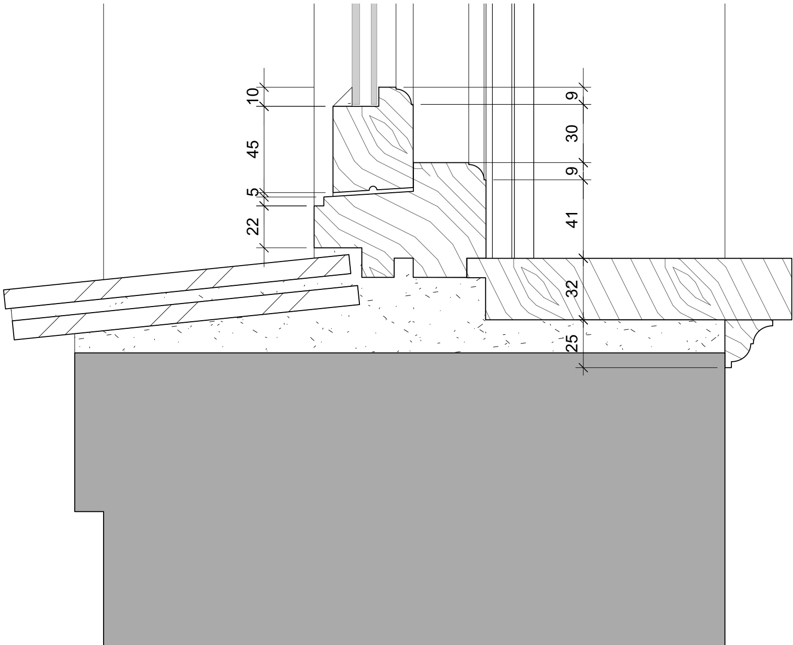
A 706.4 - SILL SCALE 1:2
