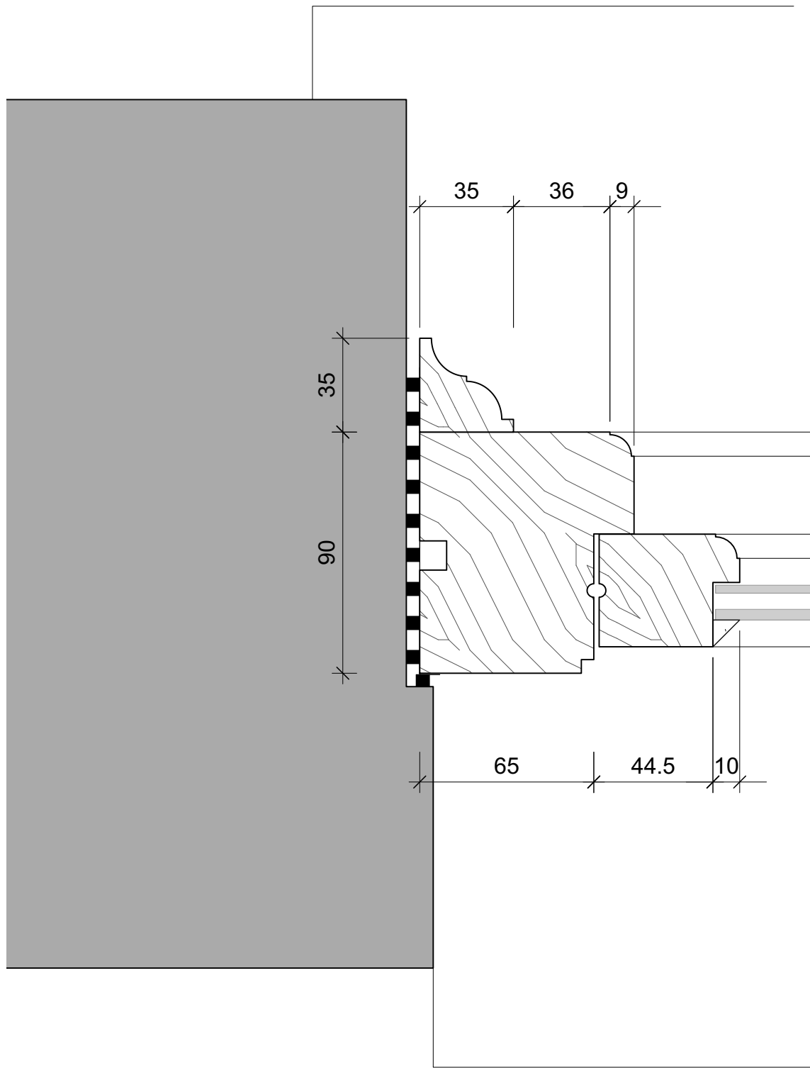
A 706.5 - JAMB SCALE 1:2
