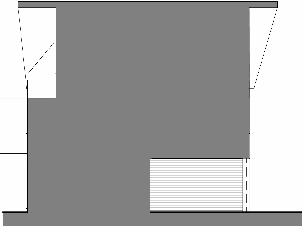
ELEVATION 3 1 : 100
