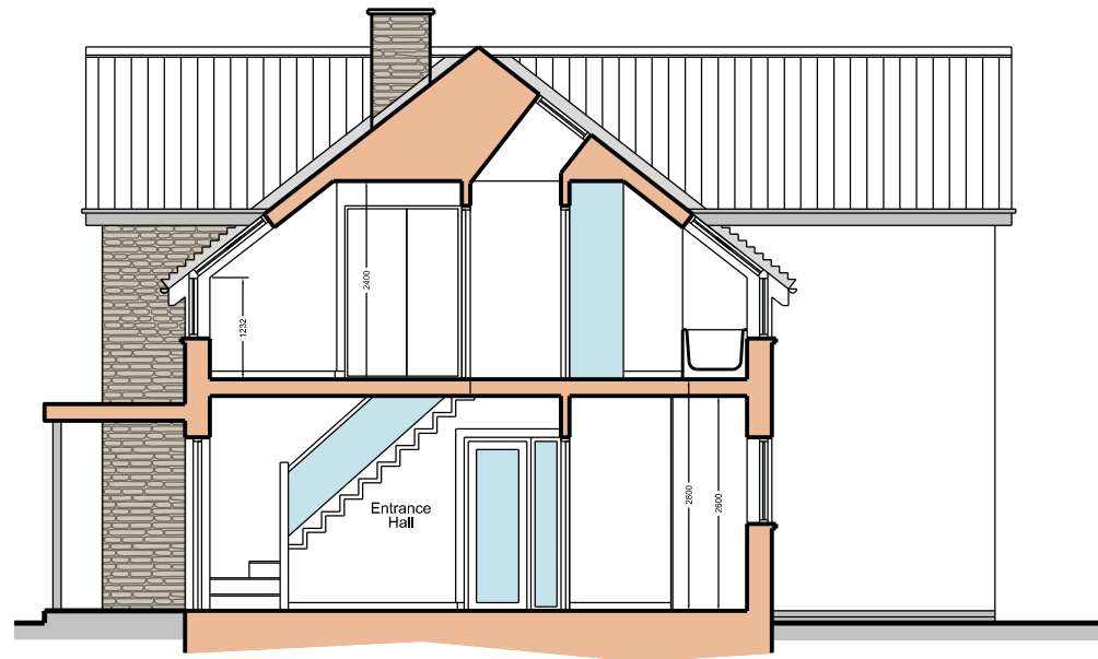
Section A - 1:100 @ A3
