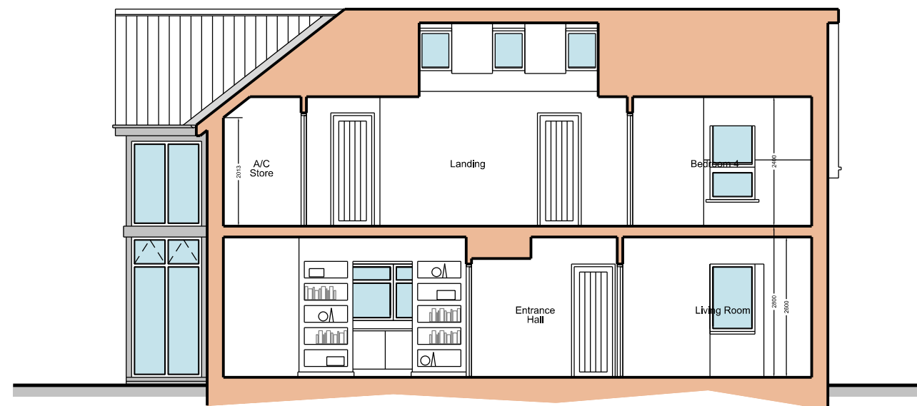
Section C - 1:100 @ A3
