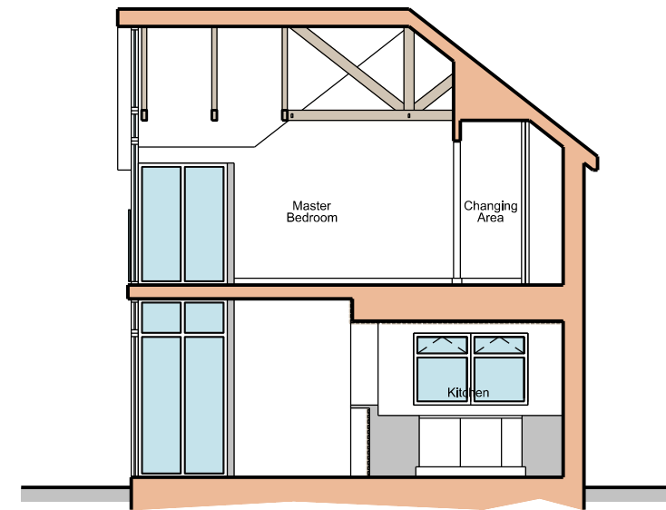
Section B - 1:100 @ A3
