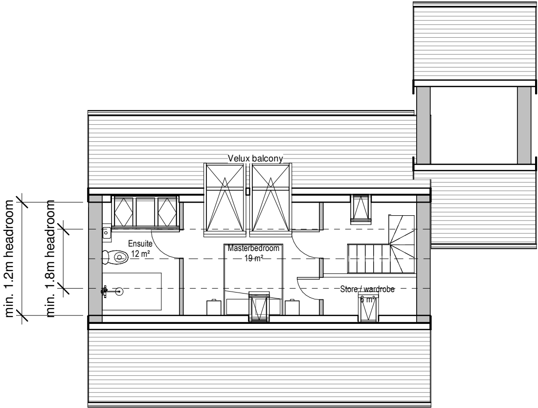
New Loft floor ( 1 : 100)
