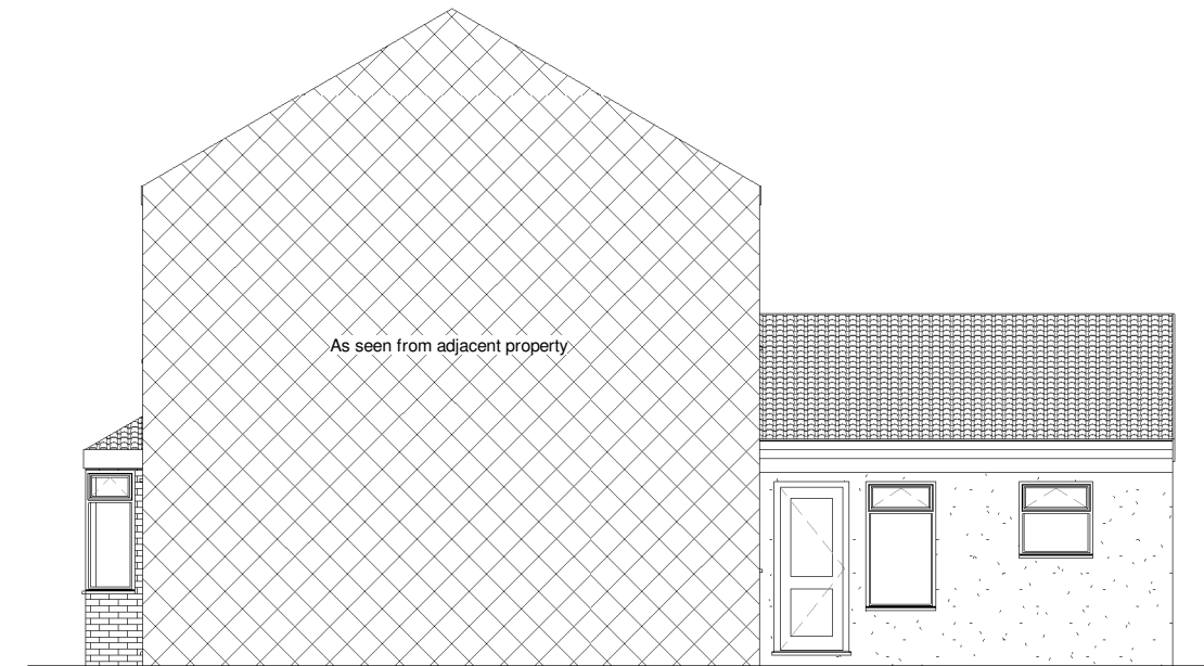
Right Elevation 1 : 100
