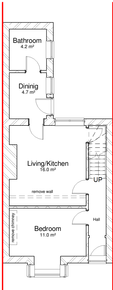
GF 1 : 100
