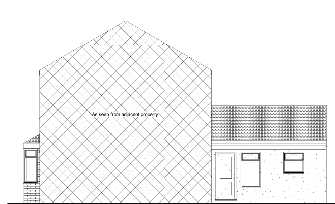
Right Elevation 1 : 100
