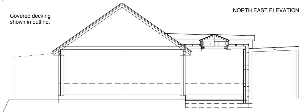
DIAGRAMMATIC SECTION AA.
