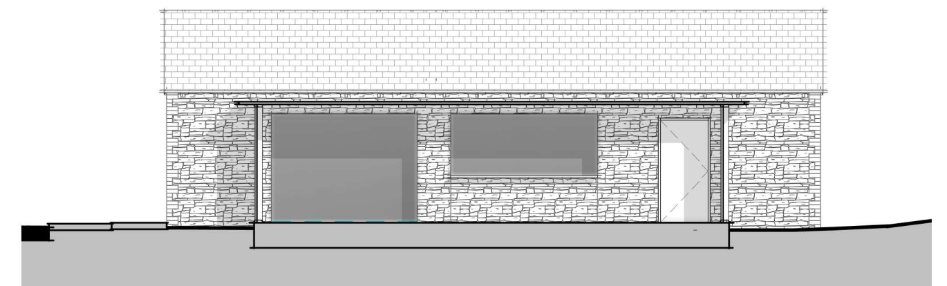
6 Section B_B 1 : 100
