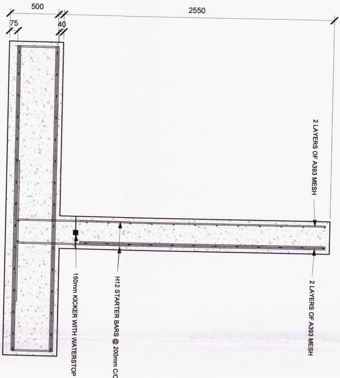
3 REBAR DETAIL 1 : 20
