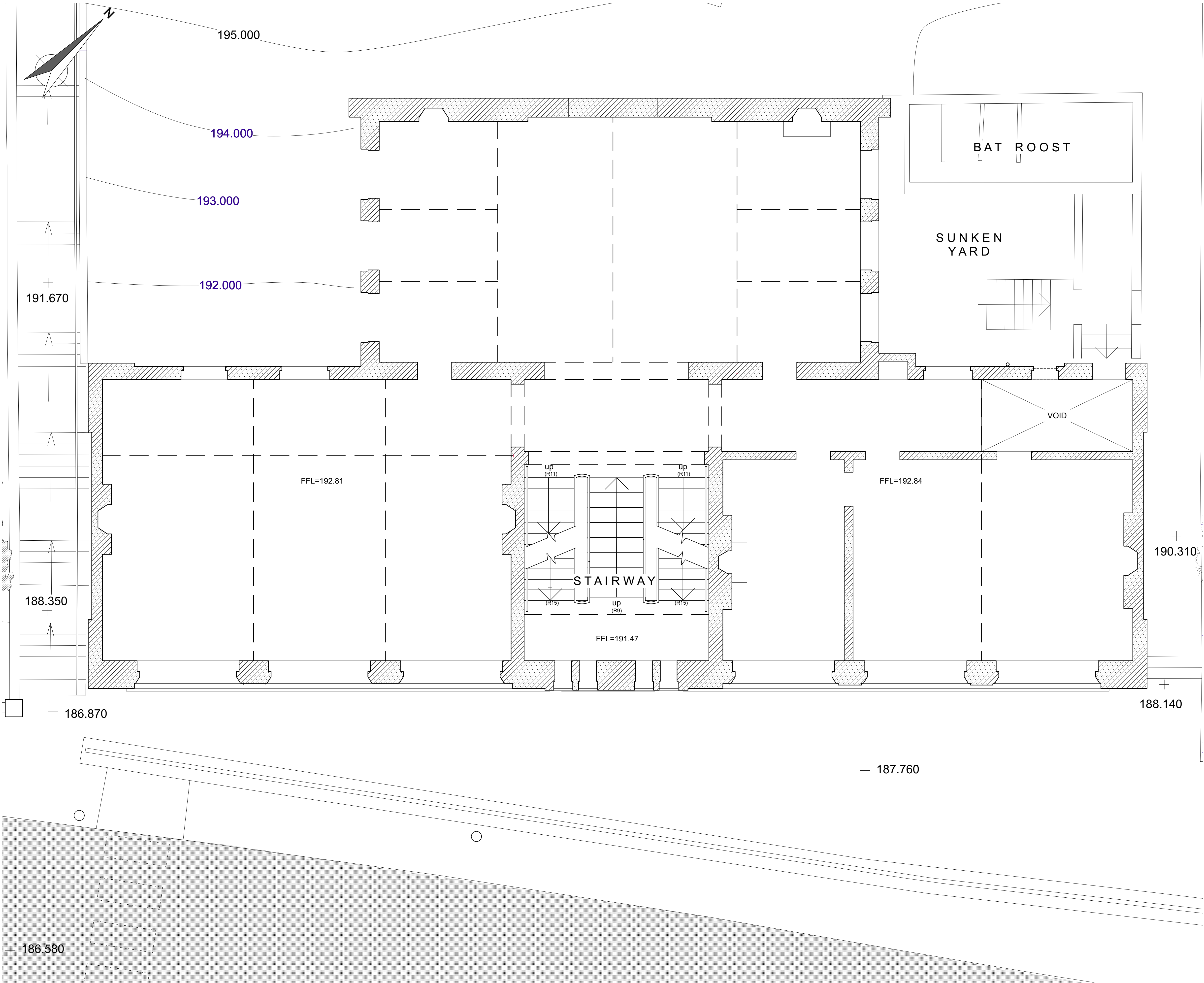
1 Mezzanine Demolition Plan Scale: 1:50
