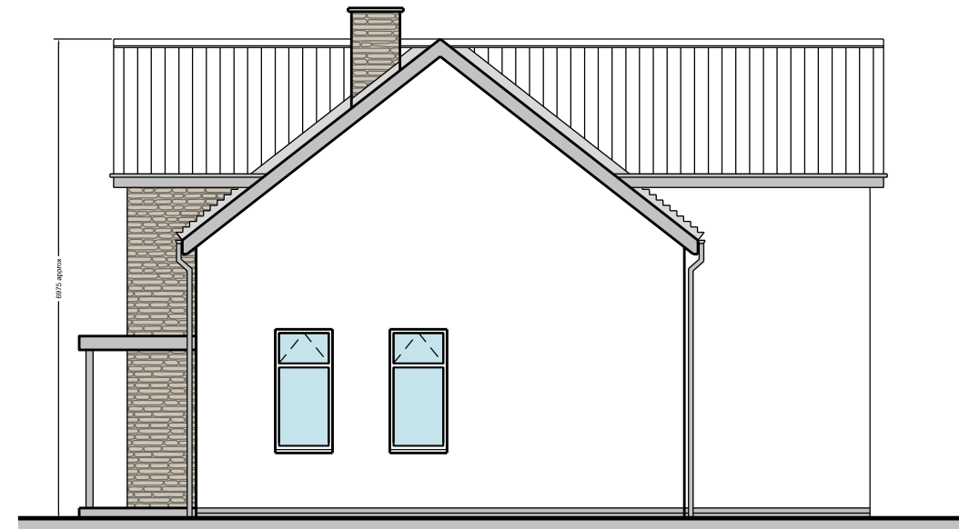
Side Elevation - 1:100 @ A3
