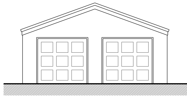
EXISTING SE ELEVATION
