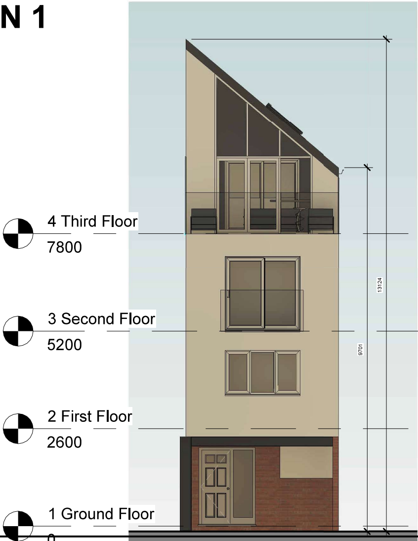
ELEVATION 4 1 : 100
