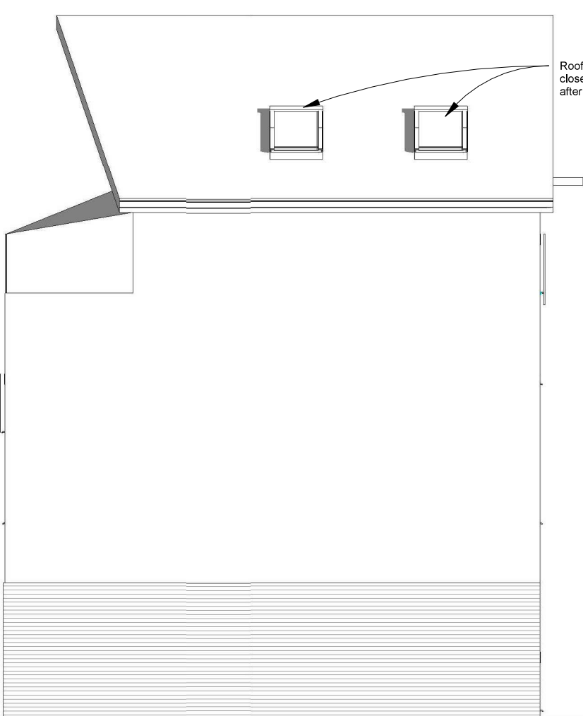
ELEVATION 2 1 : 100
