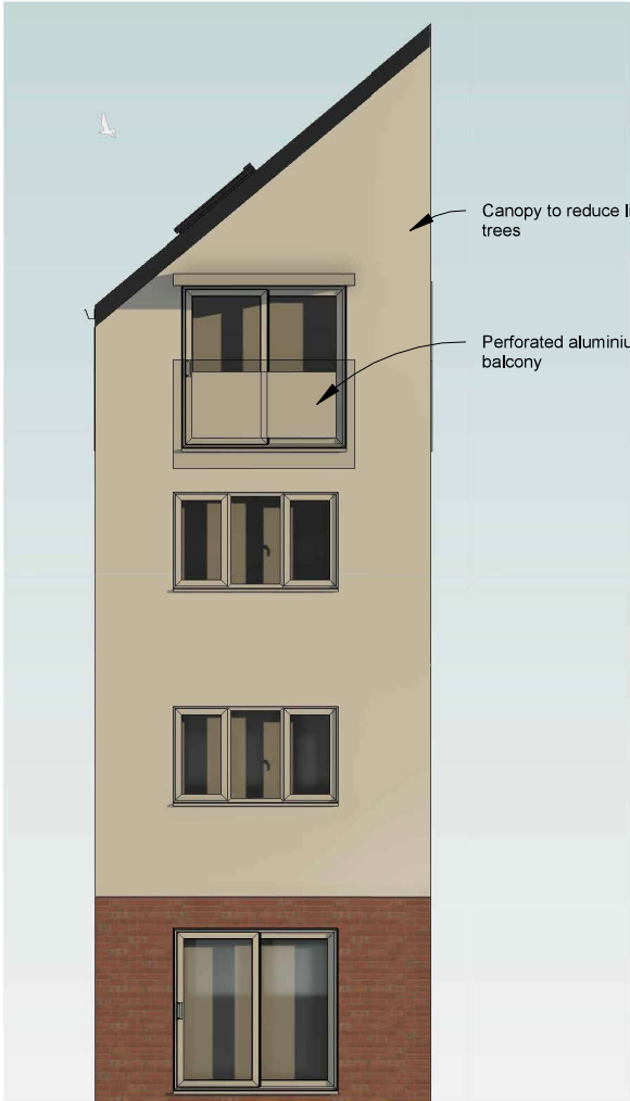
ELEVATION 1 1 : 100
