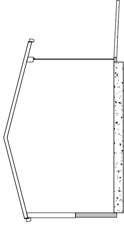
6 Existing Section 1 : 100
