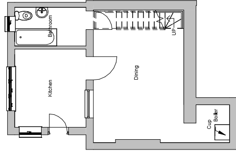
⑤ Existing Basement 1 : 100
