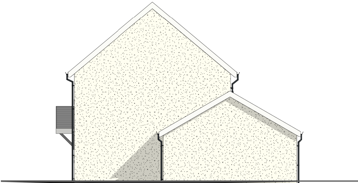
North Elevation ( 1 : 100)
