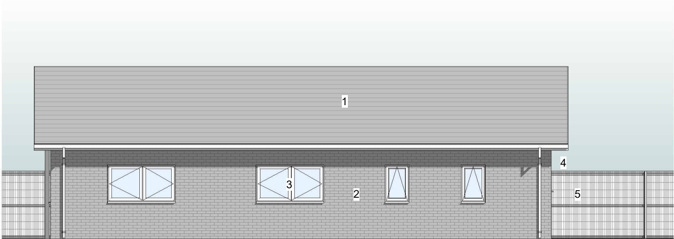
West Existing ( 1 : 100)
