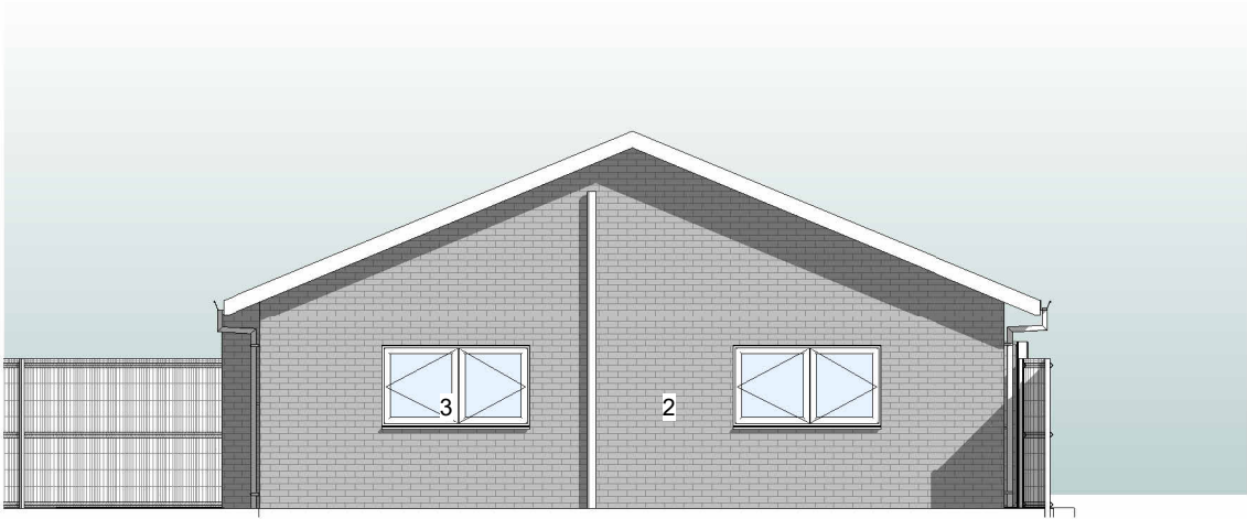
North Existing ( 1 : 100)
