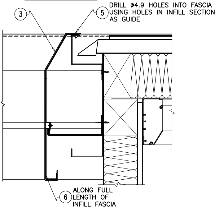
SECTION 'B-B'
