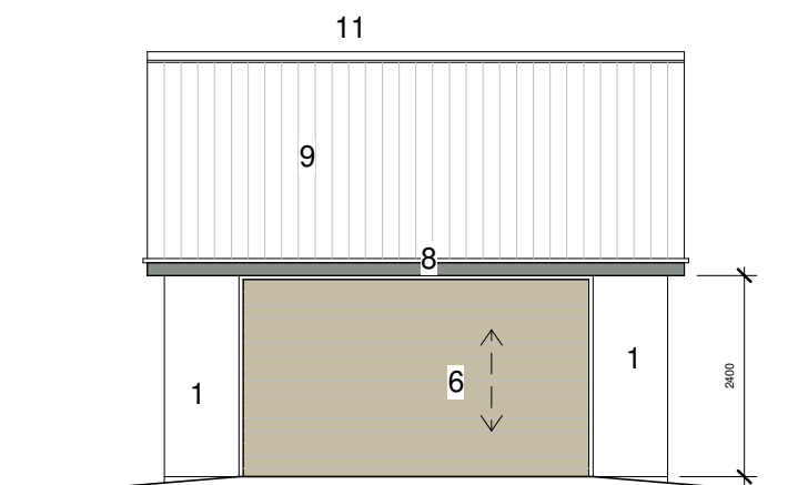
Front Elevation - 1:100 @ A3
