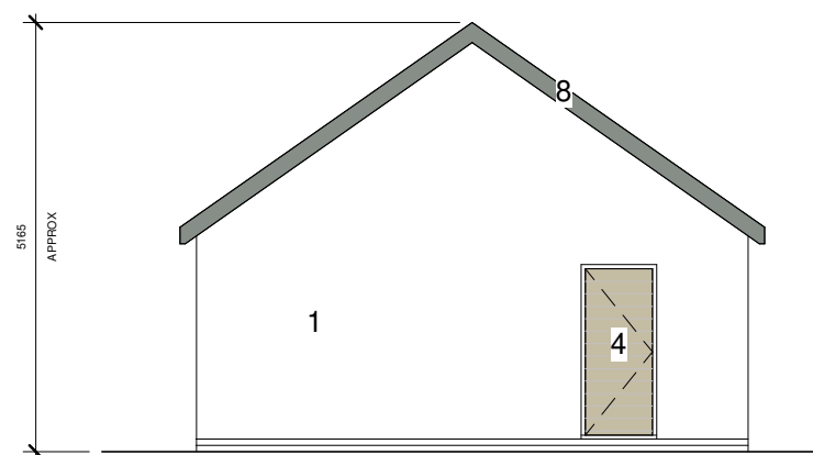
Side Elevation - 1:100 @ A3
