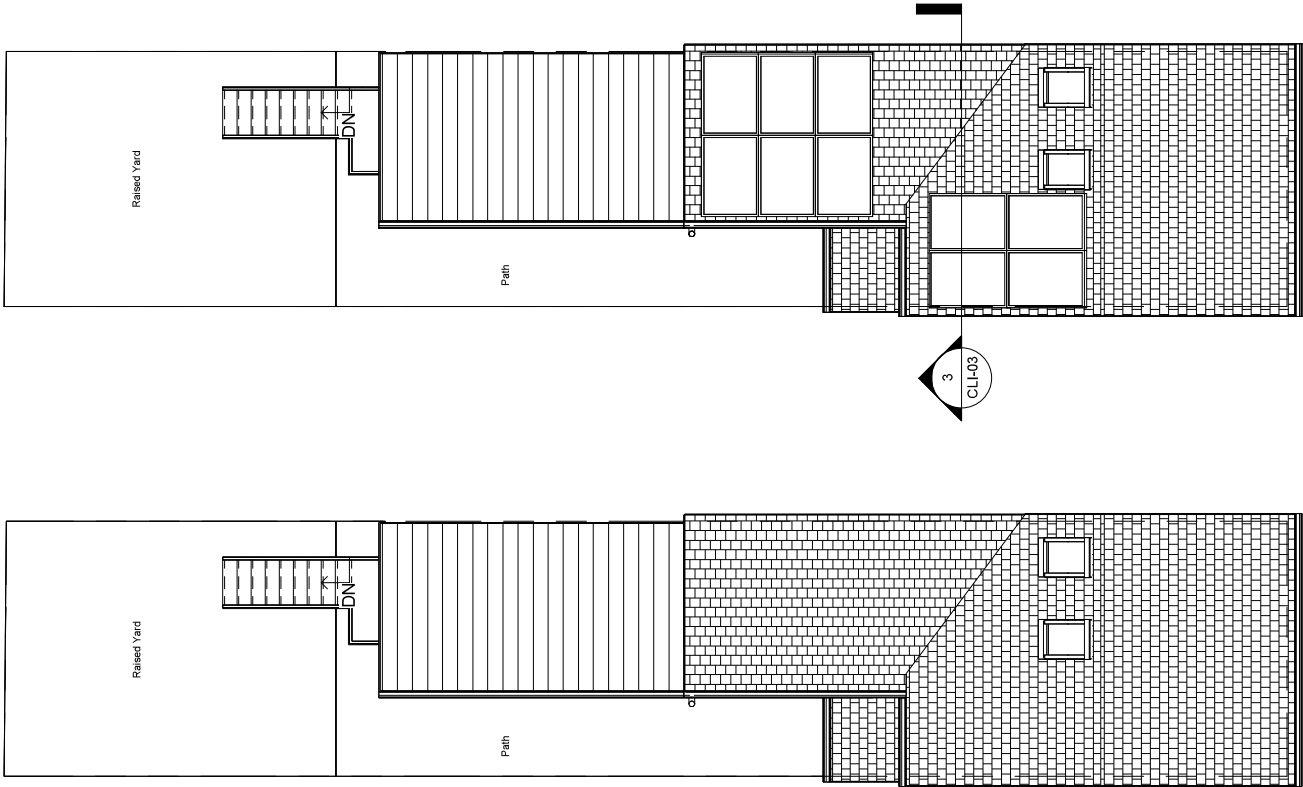
1 Existing Site 1 : 100
