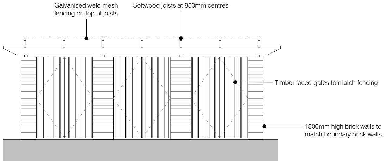
Elevation A
